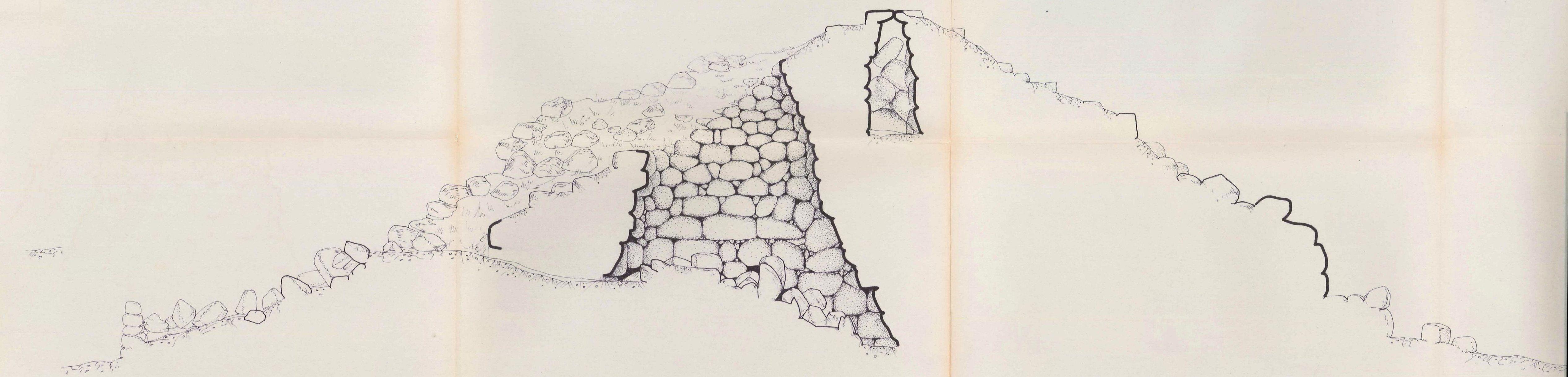
sezione c-d
